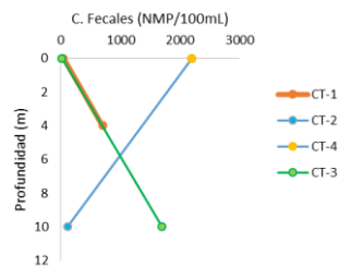
Fig. 4: Perfil de estaciones realizadas en la transecta de Noviembre de 2015 en la ensenada de Tortel (Fig.3).
